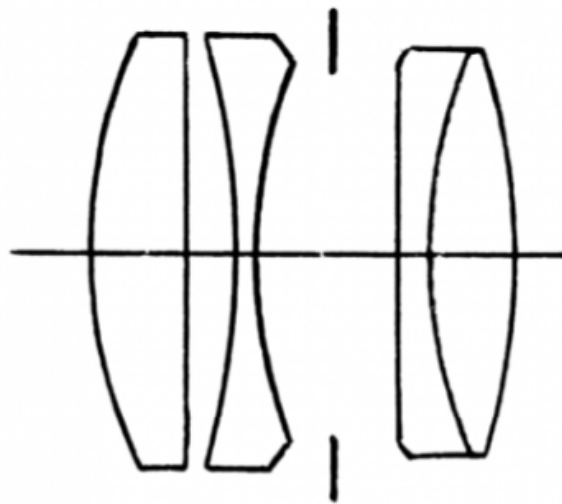
Figure 6.6. The Zeiss Tessar.
